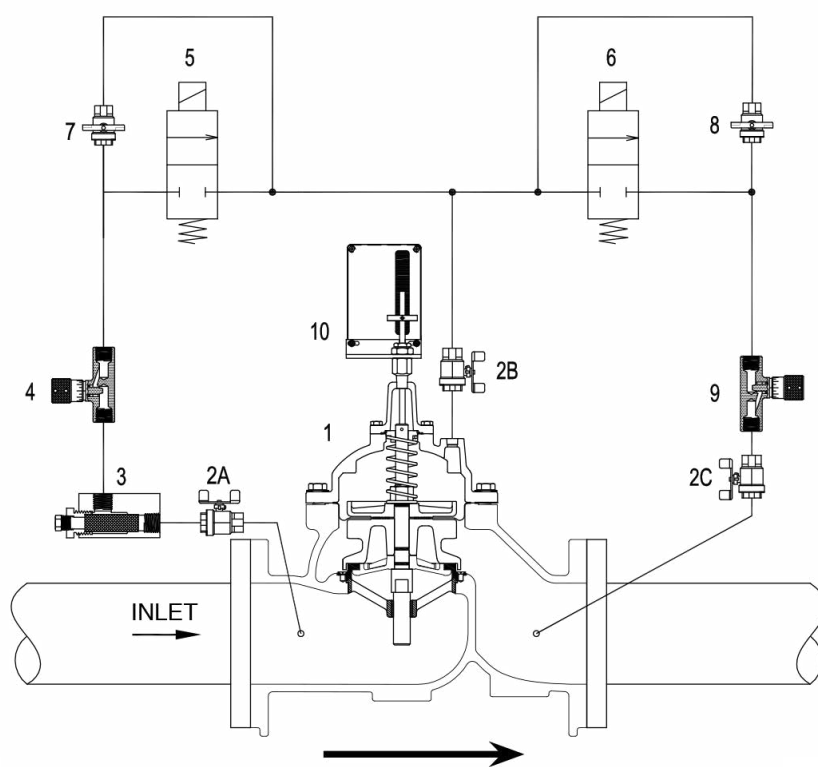
FIG. 2 Schematic A-7637A
