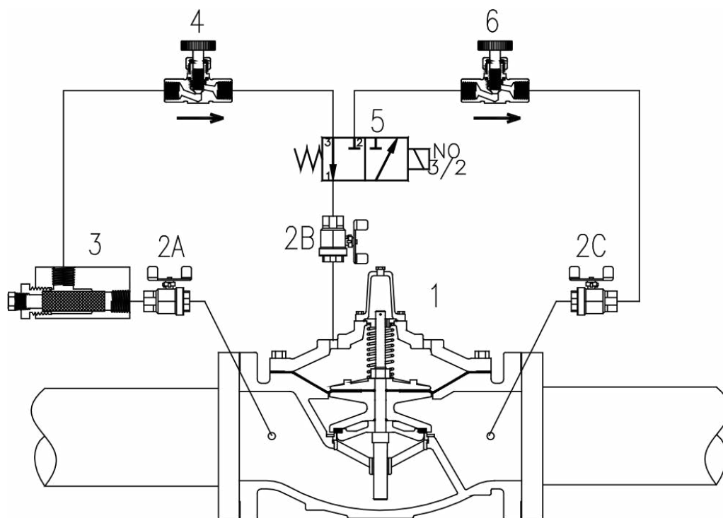
FIG. 2 Schematic A-0593C
