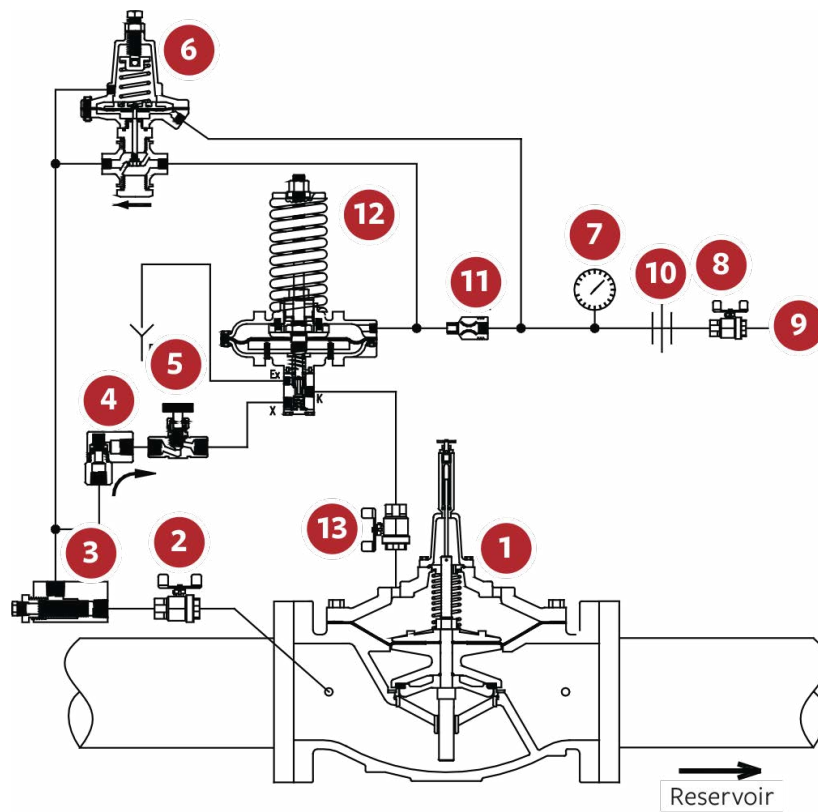
SCHEMATIC A-04140
